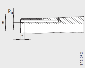
液压紧定套（后缀为 HG） 安装尺寸
