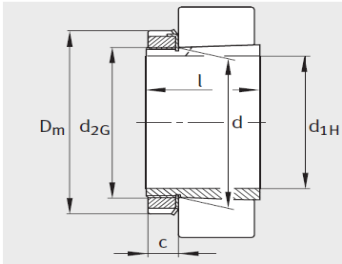
锥度为 1：12（H240、H241 系列，锥度为 1：30） 止动垫圈 MB、MBL
