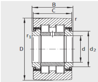
PWTR...-2RS ( 优化的 INA 轮廓形状 )
