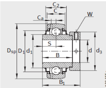
GE...KRR-B、E...KRR-B、 GE...KLL-B
