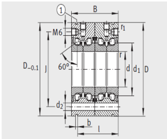
ZKLF-2RS-2AP ① 拉拔槽
