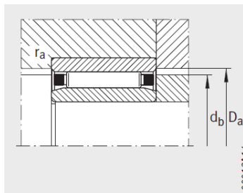
滚针和保持架组件 在轴上的轴向引导
